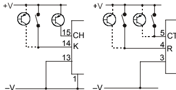
Entrada tipo Source (PNP)
