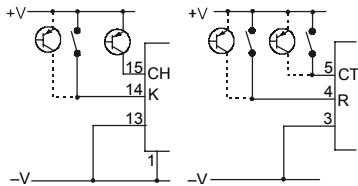
Source (PNP) Inputs
