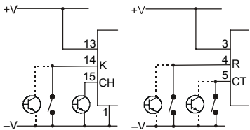
Sink (NPN) Inputs
