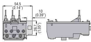
G244 button
