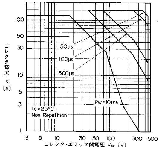
安全動作領域特性(非線返し)
