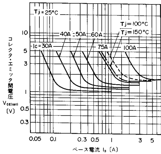
出力特性
