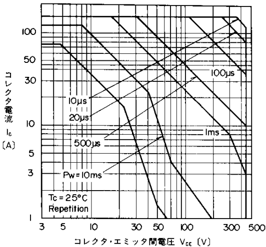
安全動作領域特性(線返し)
