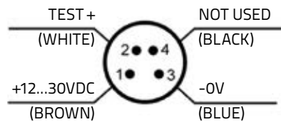
EMITTER G
