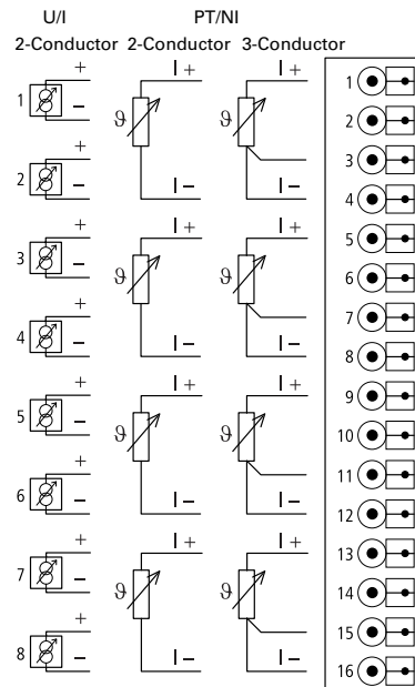
XNE-8AI-U/I-4PT/NI
