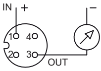
1 (IN) 3 (OUT)
