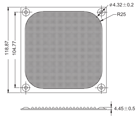
FM 12 For 120mm Fan
