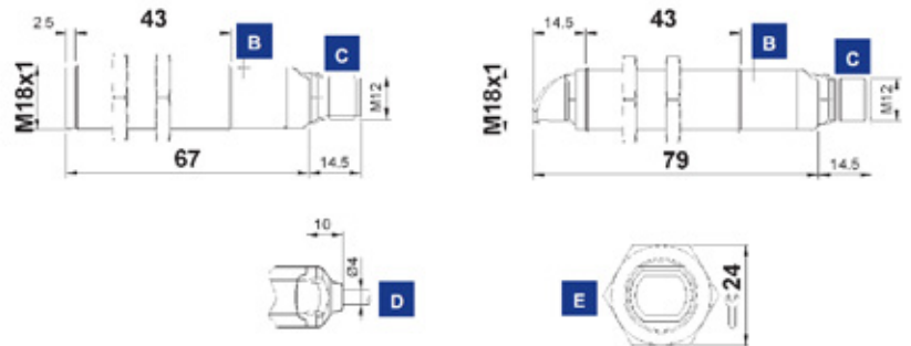
CONTENITORE METALLICO
