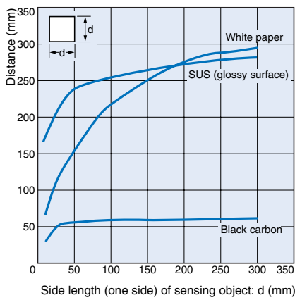
Diffuse-reflective E3Z-D□1(D□6)
