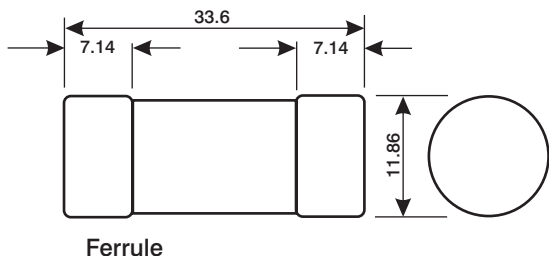
Ferrule
